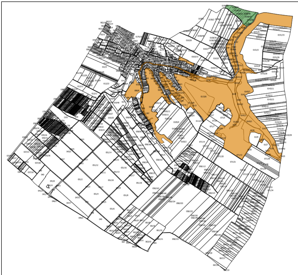
Az ökológiai hálózat magterületének és az ökológiai hálózat ökológiai folyosójának lehatárolása az adatszolgáltatás alapján
